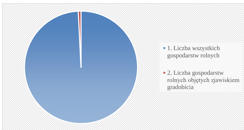
Wykres 9: Zjawisko deszczu nawalnego i huraganu na terenie gminy
