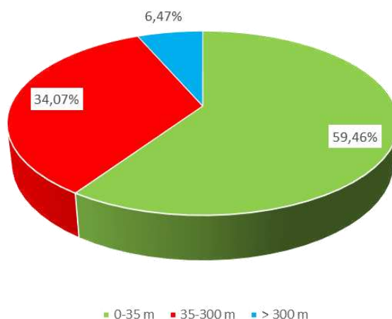
Rys. nr 19. Udział procentowy ptaków w odniesieniu do trzech pułapów wysokości (poniżej, powyżej i w zasięgu łopaty wirnika)
