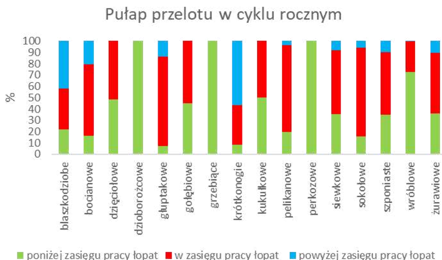
Rys. nr 20. Pułapy przelotów ptaków w cyklu rocznym
