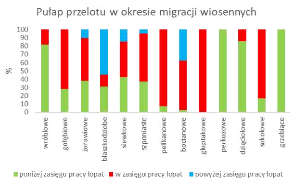
Rys. nr 21. Pułapy przelotów ptaków w okresie migracji wiosennej
