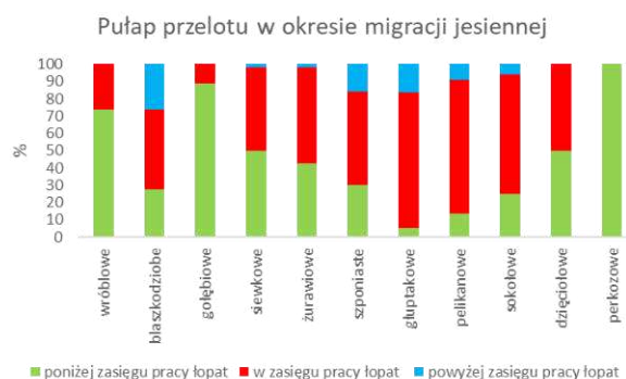
Rys. nr 24. Pułapy przelotów ptaków w okresie migracji jesiennej
