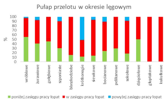
Rys. nr 22. Pułapy przelotów ptaków w okresie lęgowym
