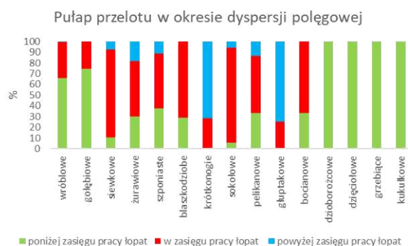
Rys. nr 23. Pułapy przelotów ptaków w okresie dyspersji połęgowej
