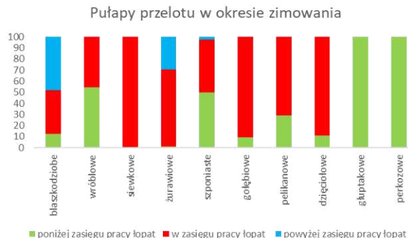
Rys. nr 25. Pułapy przelotów ptaków w okresie zimowania
